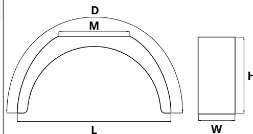
Parafango sommità piatta rotazionale Rotational flat top mudguard
