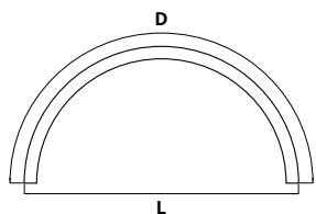
Parafanghi termoplastici ad iniezione Mudguards injection moulding
